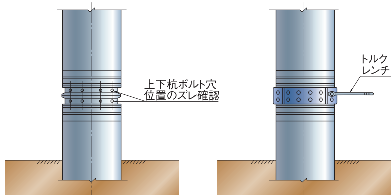
2 上杭を下杭に垂直に載せる (ガイドピン(凹凸)を合わせ ながら載せる)
