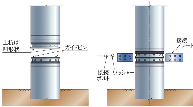
1 下杭端板に接続ボルト位置 合わせ用ガイドピン取付 (上杭端板は凹形状)
