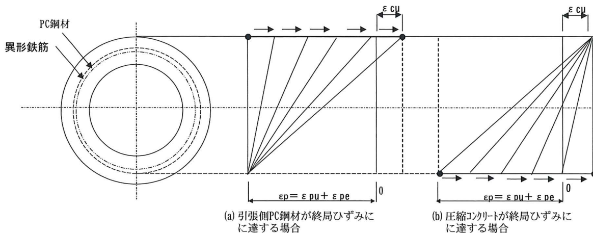
図 1 1 - 4 破壊時のひずみ図
