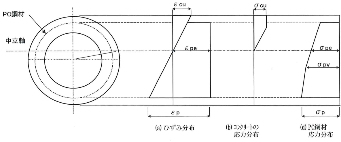
図 1 1 - 5 破壊時のひずみおよび応力分布図
