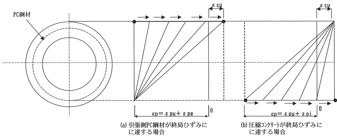
図 1 1 - 6 破壊時のひずみ図
